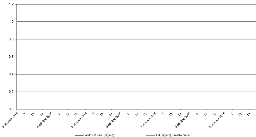
Metano - CH 4 Stazione di rilevamento di via B. Cairoli, periodo: 03 ott 2016 - 09 ott 2016
