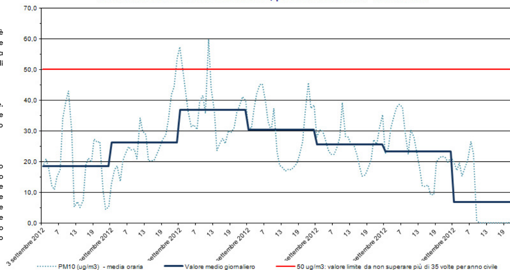
PM 10 Stazione di rilevamento di via B. Cairoli, periodo: 03 set 2012 - 09 set 2012
