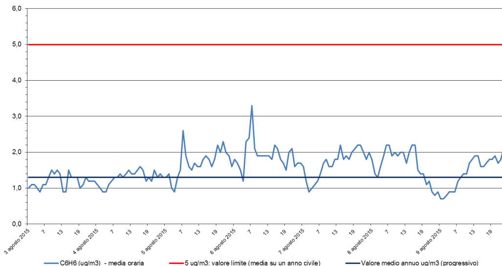
Benzene - C 6 H 6 Stazione di rilevamento di Sambruson, periodo: 03 ago 2015 - 09 ago 2015
