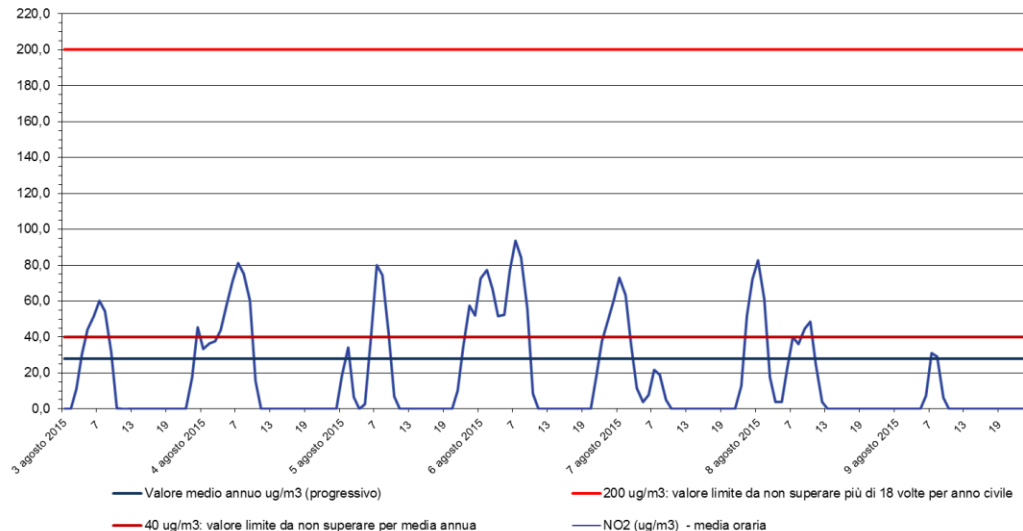
Biossido di azoto - NO 2 Stazione di rilevamento di Sambruson, periodo: 03 ago 2015 - 09 ago 2015
