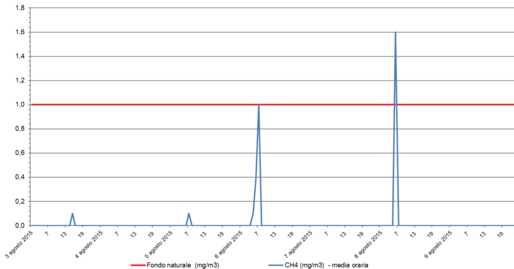
Metano - CH 4 Stazione di rilevamento di Sambruson, periodo: 03 ago 2015 - 09 ago 2015
