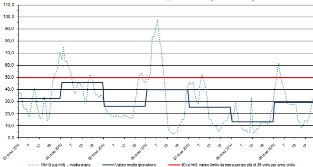
PM10 Stazione di rilevamento di via F.lli Bandiera, periodo: 03 mag 2010 - 09 mag 2010
