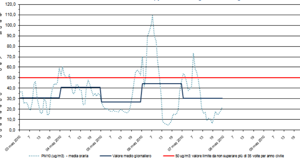
PM 10 Stazione di rilevamento di via B. Cairoli, periodo: 03 mag 2010 - 09 mag 2010
