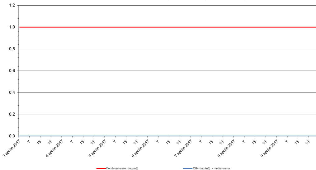
Metano - CH 4 Stazione di rilevamento di via B. Cairolì, periodo: 03 apr 2017 - 09 apr 2017
