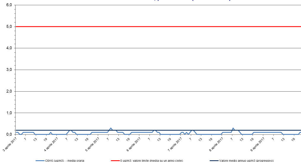
Benzene - C 6 H 6 Stazione di rilevamento di Sambruson, periodo: 03 apr 2017 - 09 apr 2017
