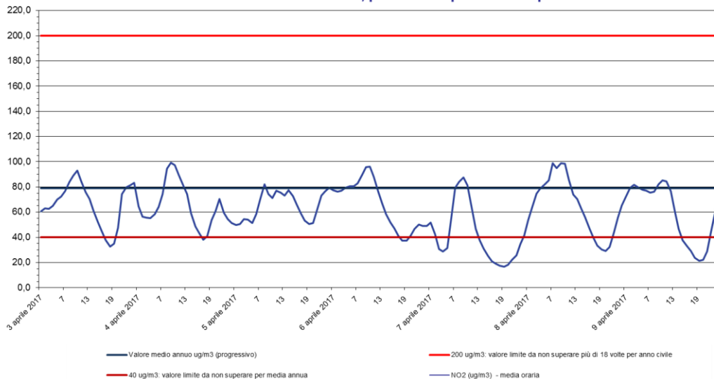
Biossido di azoto - NO 2 Stazione di rilevamento di Sambruson, periodo: 03 apr 2017 - 09 apr 2017
