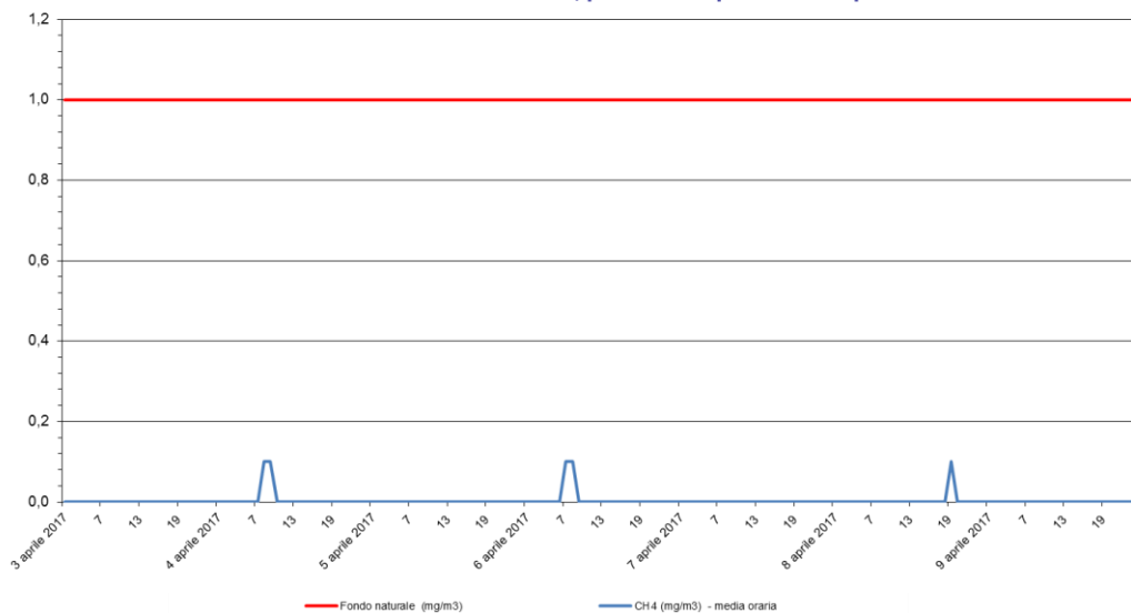
Metano - CH 4 Stazione di rilevamento di Sambruson, periodo: 03 apr 2017 - 09 apr 2017
