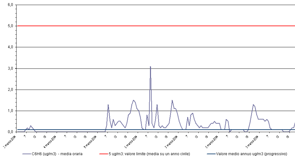
Benzene - C 6 H 6 Stazione di rilevamento di Sambruson, periodo: 03 mar 2014 - 09 mar 2014
