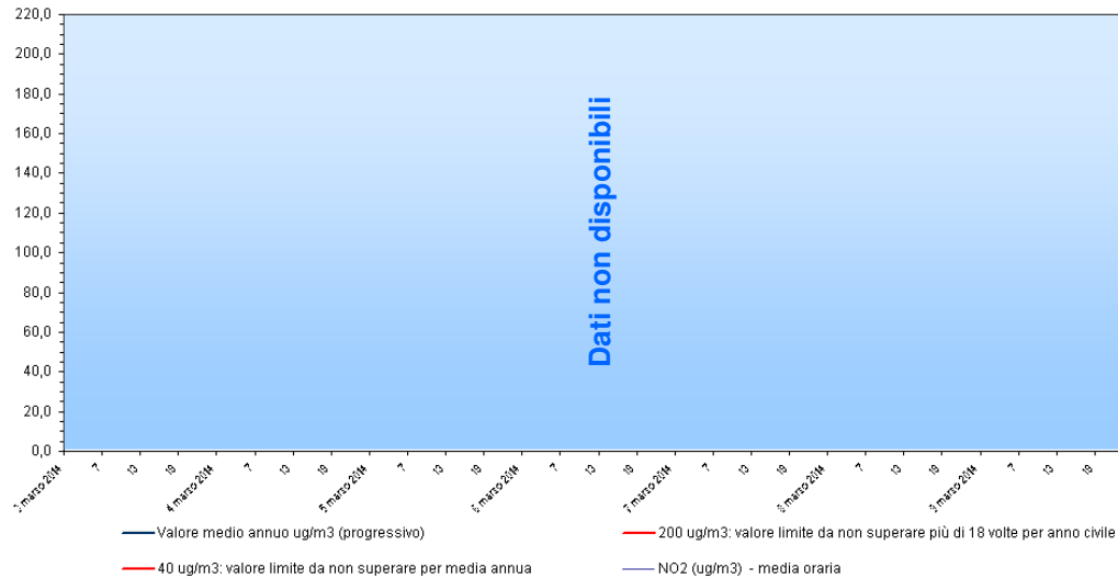
Biossido di azoto - NO 2 Stazione di rilevamento di Sambruson, periodo: 03 mar 2014 - 09 mar 2014
