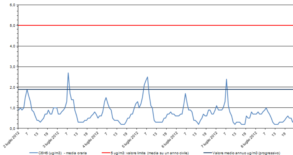
Benzene - C 6 H 6 Stazione di rilevamento di via B. Cairoli, periodo: 02 lug 2012- 08 lug 2012
