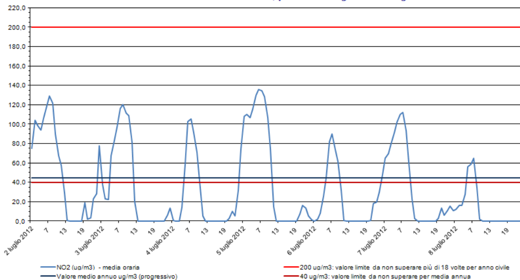
Biossido di azoto - NO 2 Stazione di rilevamento di via B. Cairoli, periodo: 02 lug 2012- 08 lug 2012
