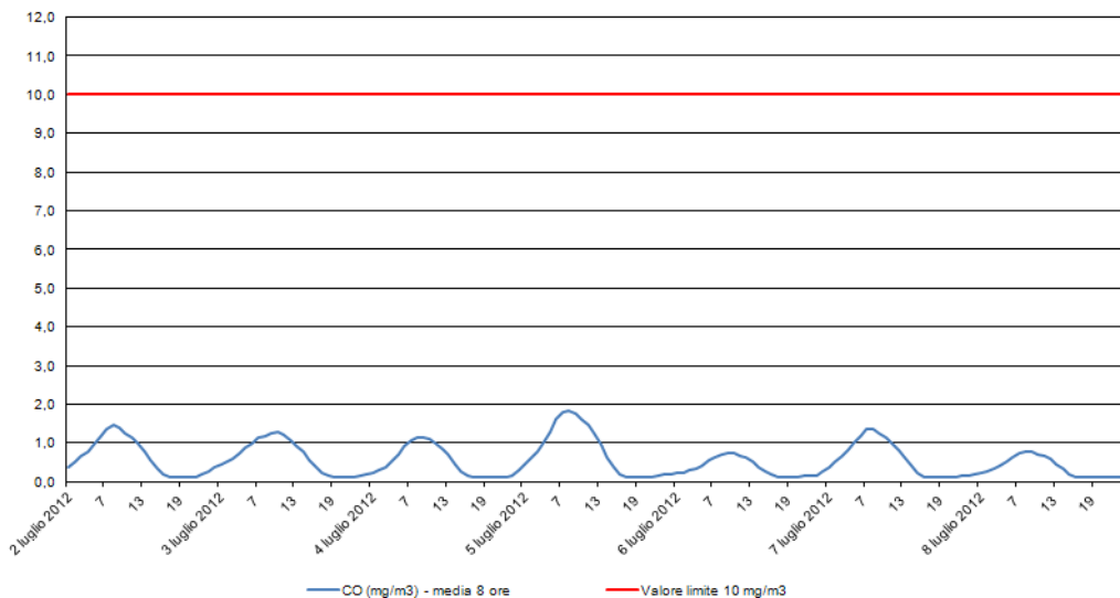
Monossido di Carbonio - CO Stazione di rilevamento di via B. Cairoli, periodo: 02 lug 2012- 08 lug 2012
