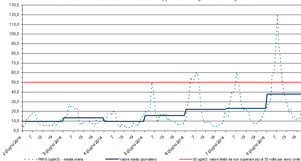
PM10 Stazione di rilevamento di via B. Cairoli, periodo: 02 giu 2014 - 08 giu 2014
