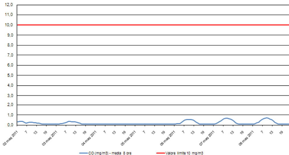
Monossido di Carbonio - CO Stazione di rilevamento di via B. Cairoli, periodo: 02 mag 2011 - 08 mag 2011
