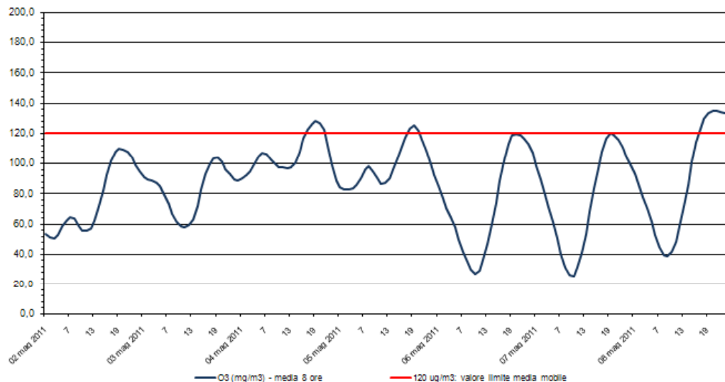
Ozono - O 3 Stazione di rilevamento di via B. Cairoli, periodo: 02 mag 2011 - 08 mag 2011
