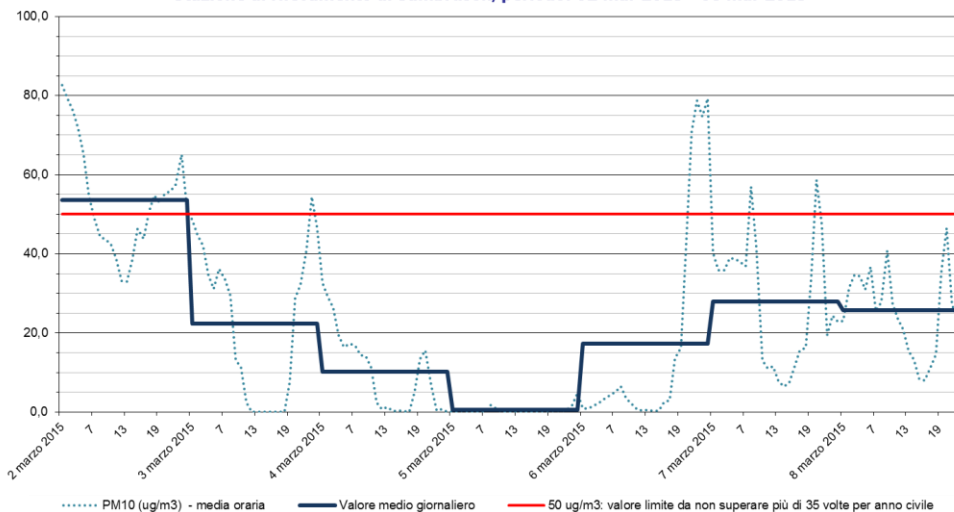
PM10 Stazione di rilevamento di Sambruson, periodo: 02 mar 2015 - 08 mar 2015
