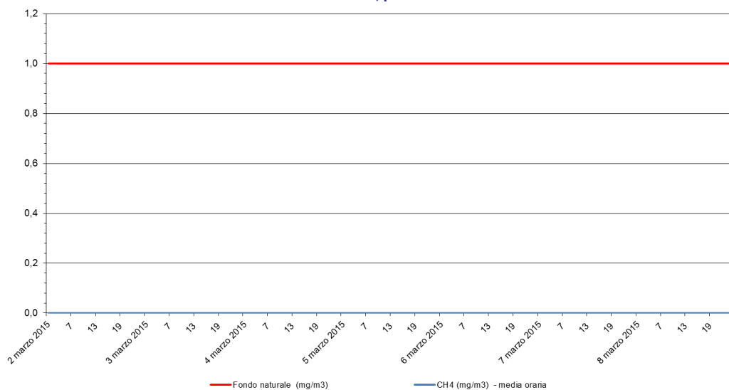
Metano - CH 4 Stazione di rilevamento di via B. Cairoli, periodo: 02 mar 2015 - 08 mar 2015
