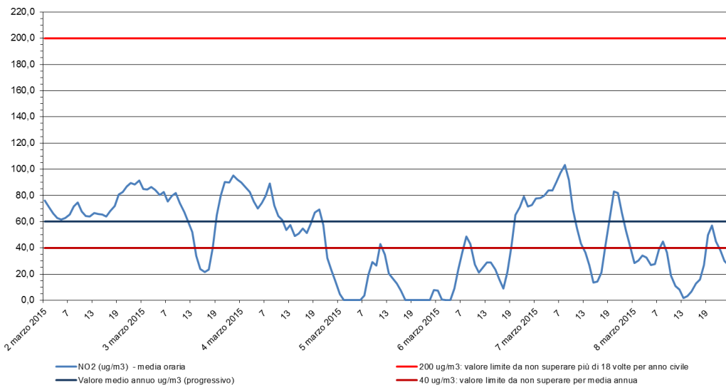
Biossido di azoto - NO 2 Stazione di rilevamento di via B. Cairoli, periodo: 02 mar 2015 - 08 mar 2015
