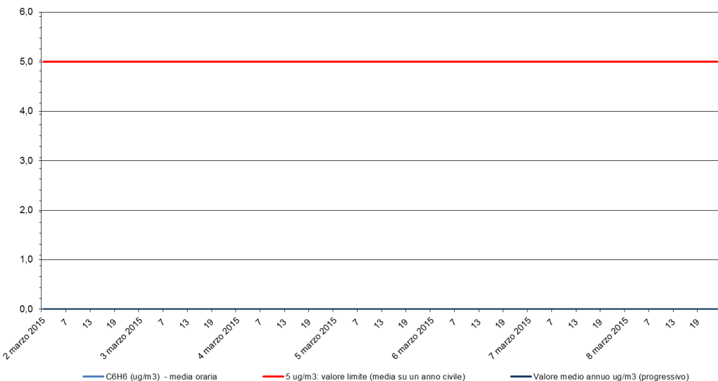
Benzene - C 6 H 6 Stazione di rilevamento di via B. Cairoli, periodo: 02 mar 2015 - 08 mar 2015
