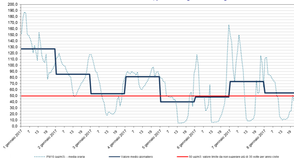
PM10 Stazione di rilevamento di via B. Cairoli, periodo: 01 gen 2017 - 08 gen 2017
