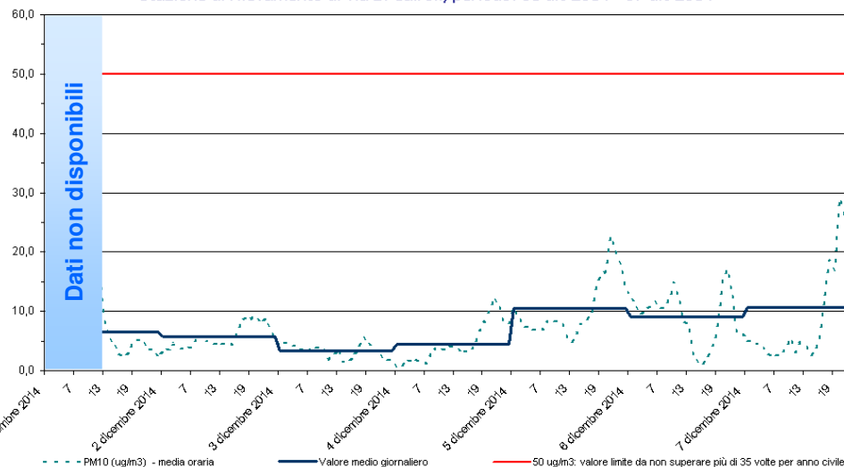
PM10 Stazione di rilevamento di via B. Cairoli, periodo: 01 dic 2014 - 07 dic 2014
