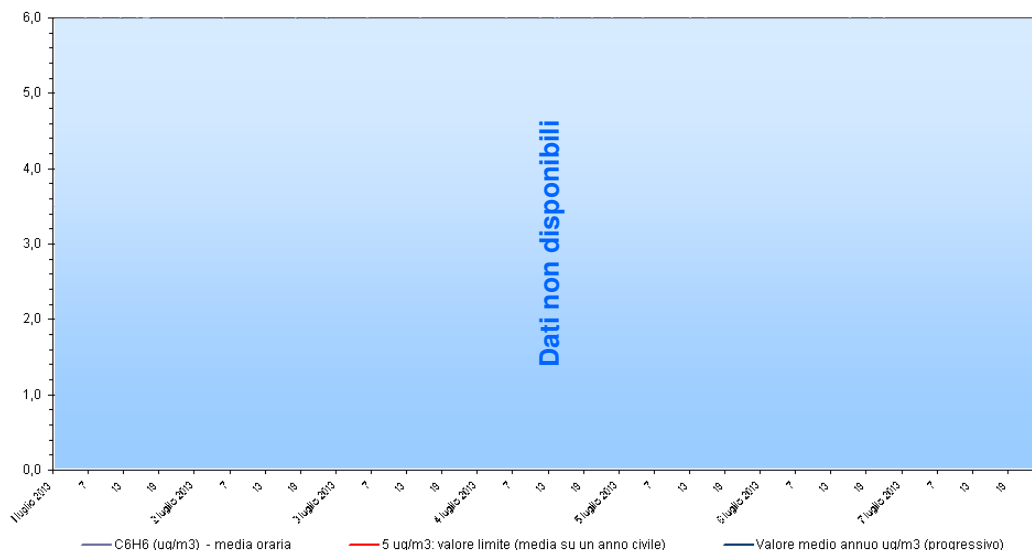
Benzene - C 6 H 6 Stazione di rilevamento di Sambruson, periodo: 01 lug 2013 - 07 lug 2013
