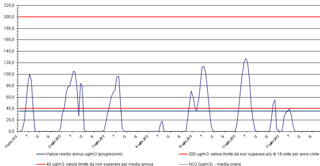
Biossido di azoto - NO 2 Stazione di rilevamento di Sambruson, periodo: 01 lug 2013 - 07 lug 2013
