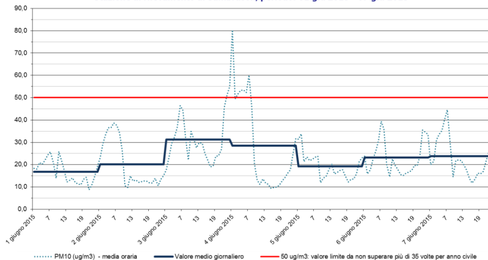
PM10 Stazione di rilevamento di Sambruson, periodo: 01 giu 2015 - 07 giu 2015
