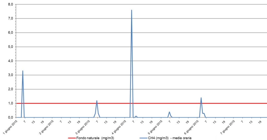
Metano - CH 4 Stazione di rilevamento di Sambruson, periodo: 01 giu 2015 - 07 giu 2015
