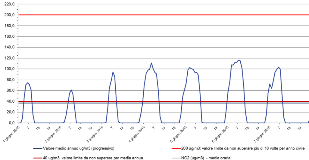
Biossido di azoto - NO 2 Stazione di rilevamento di Sambruson, periodo: 01 giu 2015 - 07 giu 2015
