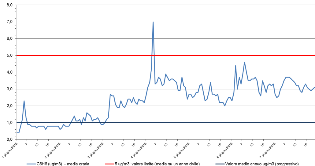
Benzene - C 6 H 6 Stazione di rilevamento di Sambruson, periodo: 01 giu 2015 - 07 giu 2015
