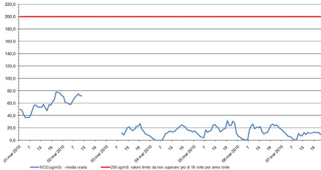
Biossido di azoto - NO 2 Stazione di rilevamento di via B. Cairoli, periodo: 01 mar 2010 - 07 mar 2010
