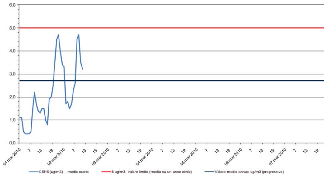
Benzene - C 6 H 6 Stazione di rilevamento di via B. Cairoli, periodo: 01 mar 2010 - 07 mar 2010
