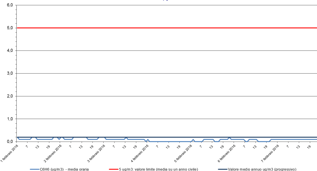
Benzene - C 6 H 6 Stazione di rilevamento di Sambruson, periodo: 01 feb 2016 - 07 feb 2016
