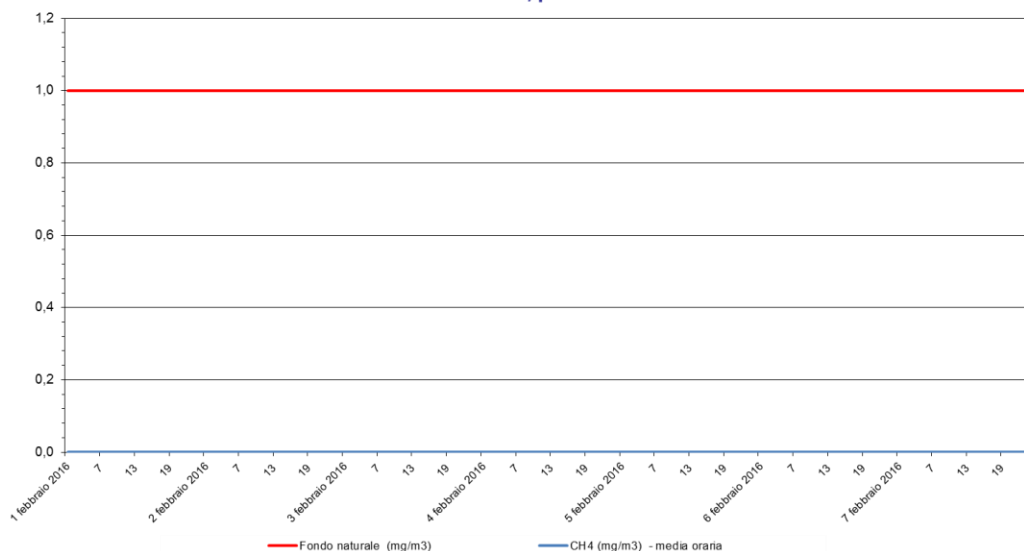
Metano - CH 4 Stazione di rilevamento di Sambruson, periodo: 01 feb 2016 - 07 feb 2016
