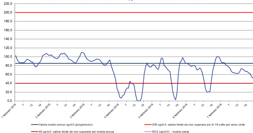
Biossido di azoto - NO 2 Stazione di rilevamento di Sambruson, periodo: 01 feb 2016 - 07 feb 2016
