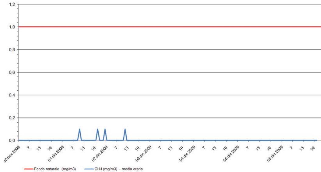
Metano - CH 4 Stazione di rilevamento di via B. Cairoli, periodo: 30 nov 2009-06 dic 2009
