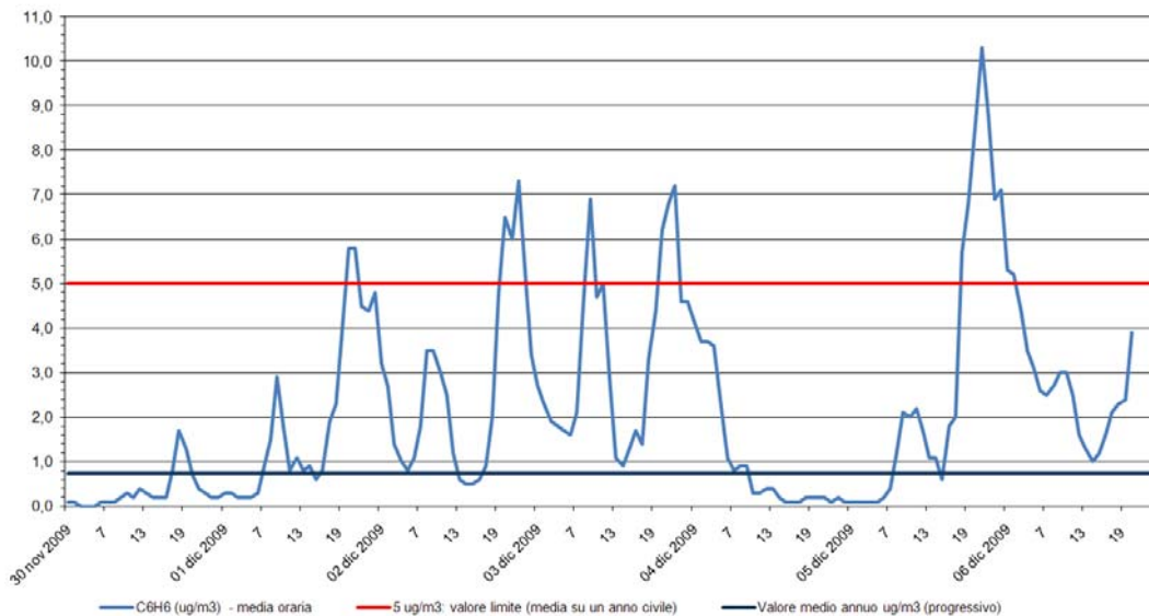
Benzene - C 6 H 6 Stazione di rilevamento di via B. Cairoli, periodo: 30 nov 2009-06 dic 2009
