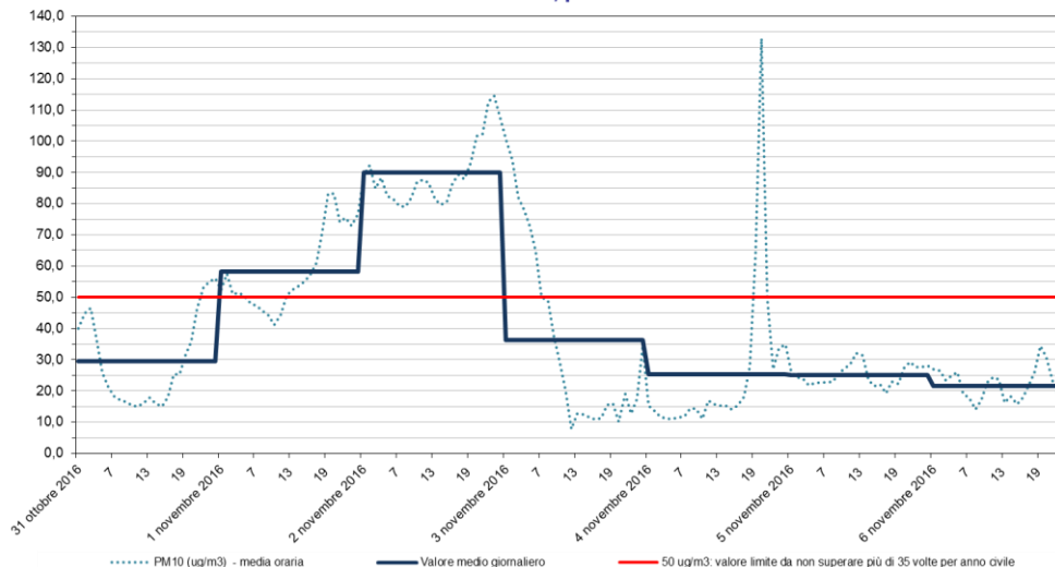
PM10 Stazione di rilevamento di via B. Cairoli, periodo: 31 ott 2016 - 06 nov 2016
