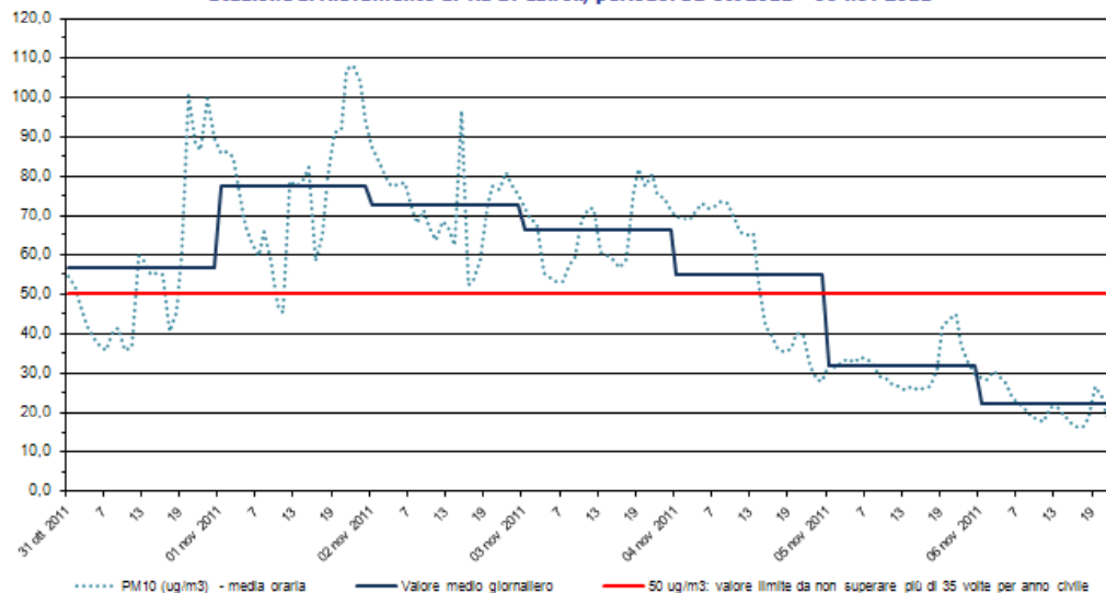
PM10 Stazione di rilevamento di via B. Cairoli, periodo: 31 ott 2011 - 06 nov 2011
