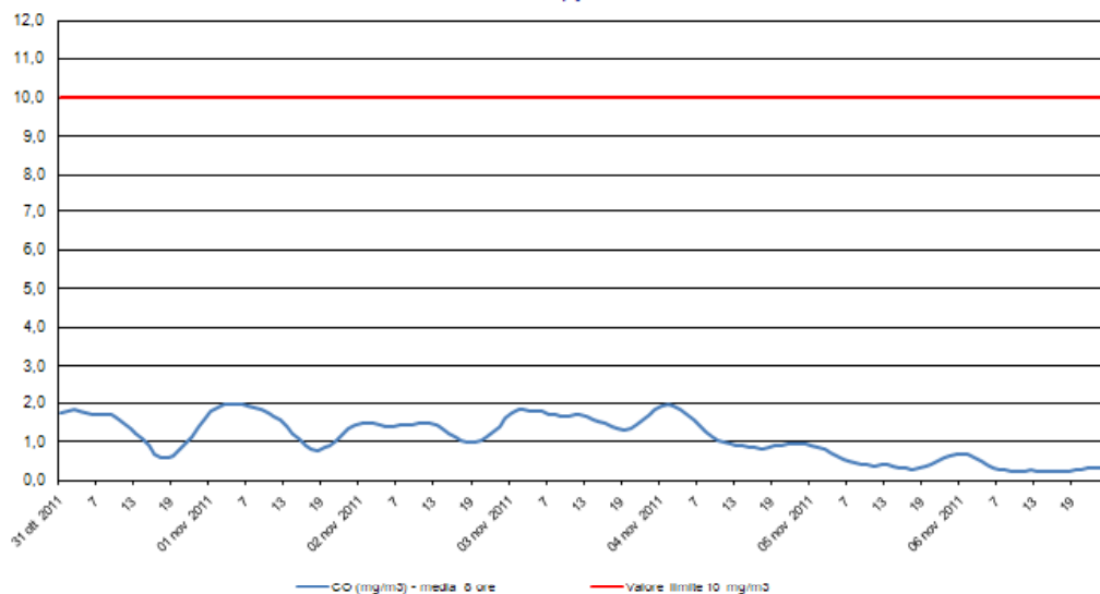
Monossido di Carbonio - CO Stazione di rilevamento di via B. Cairoli, periodo: 31 ott 2011 - 06 nov 2011
