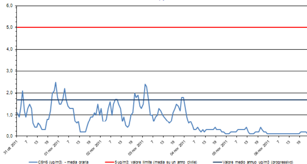
Benzene - C 6 H 6 Stazione di rilevamento di via B. Cairoli, periodo: 31 ott 2011 - 06 nov 2011
