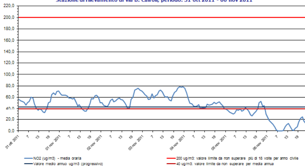
Biossido di azoto - NO 2 Stazione di rilevamento di via B. Cairoli, periodo: 31 ott 2011 - 06 nov 2011
