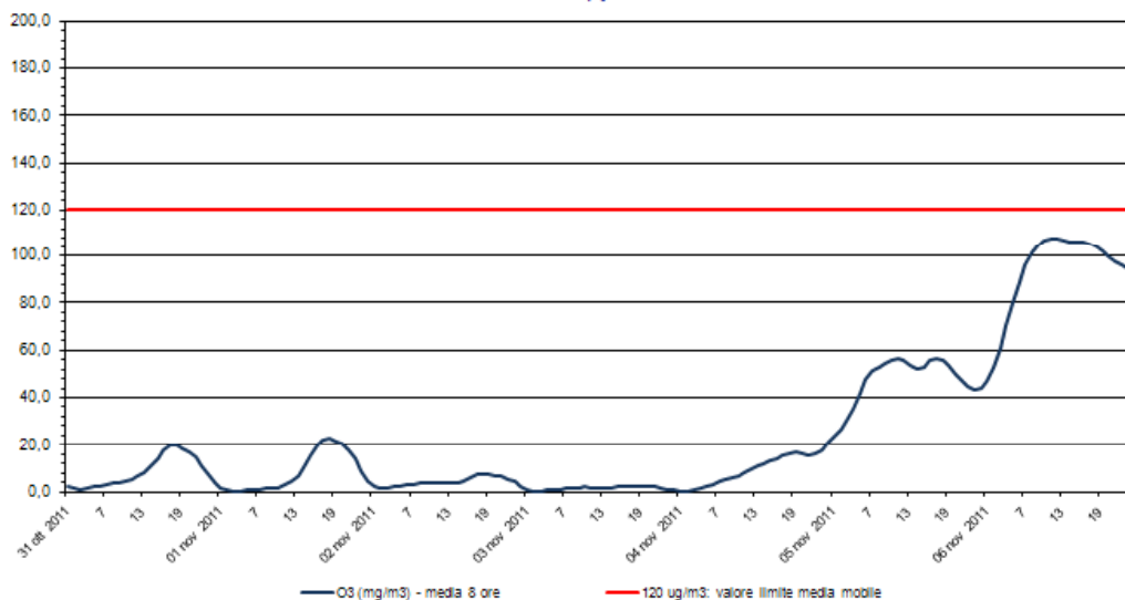
Ozono - O3 Stazione di rilevamento di via B. Cairoli, periodo: 31 ott 2011 - 06 nov 2011
