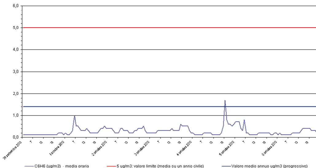
Benzene - C 6 H 6 Stazione di rilevamento di Sambruson, periodo: 30 set 2013 - 06 ott 2013
