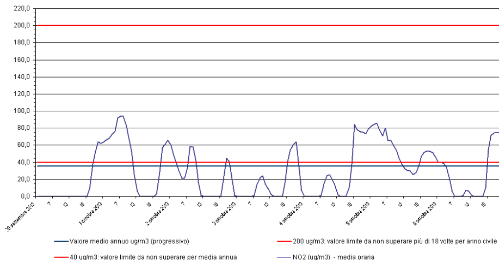
Biossido di azoto - NO 2 Stazione di rilevamento di Sambruson, periodo: 30 set 2013 - 06 ott 2013
