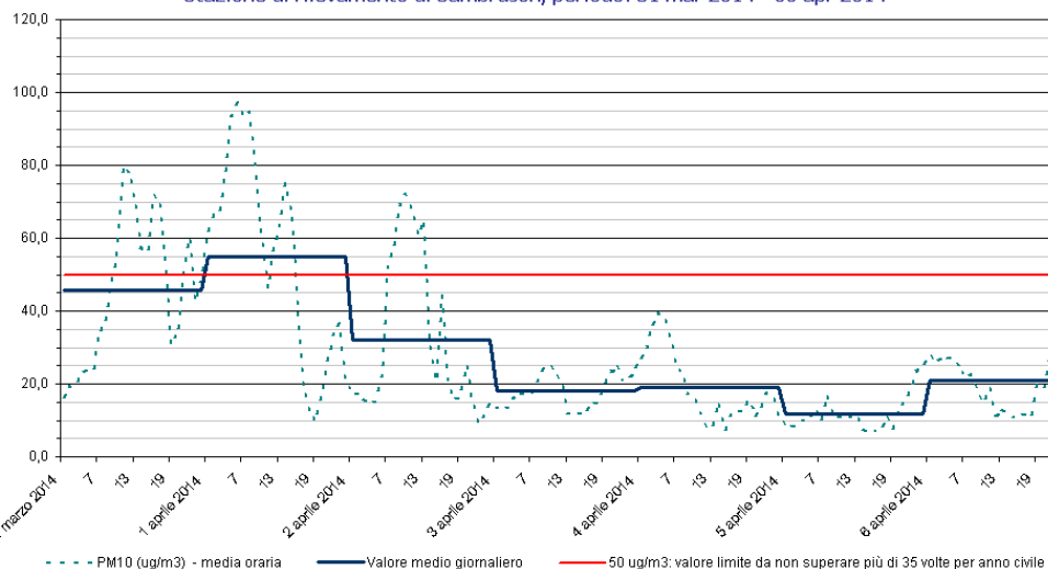
PM10 Stazione di rilevamento di Sambruson, periodo: 31 mar 2014 - 06 apr 2014
