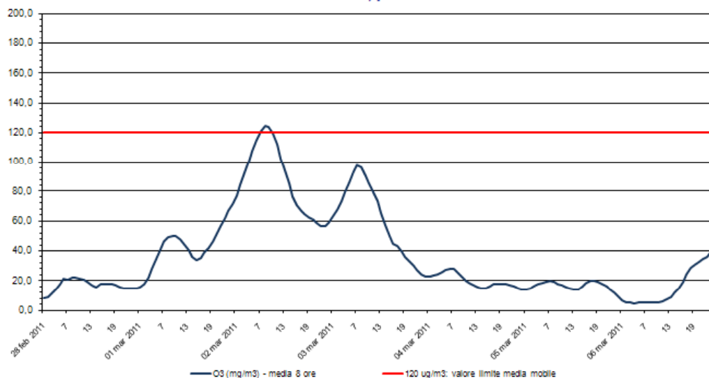
Ozono - O 3 Stazione di rilevamento di via B. Cairoli, periodo: 28 feb 2011 - 06 mar 2011
