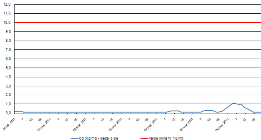
Monossido di Carbonio - CO Stazione di rilevamento di via B. Cairoli, periodo: 28 feb 2011 - 06 mar 2011
