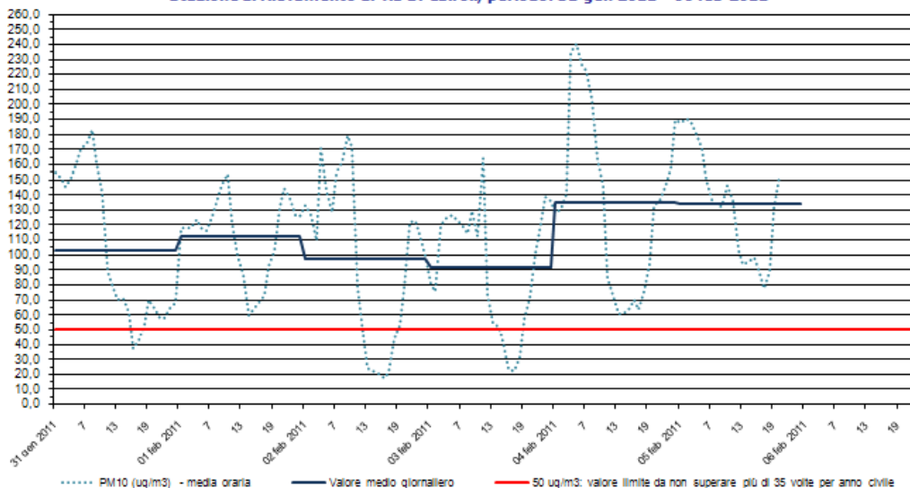
PM10 Stazione di rilevamento di via B. Cairoli, periodo: 31 gen 2011 - 06 feb 2011
