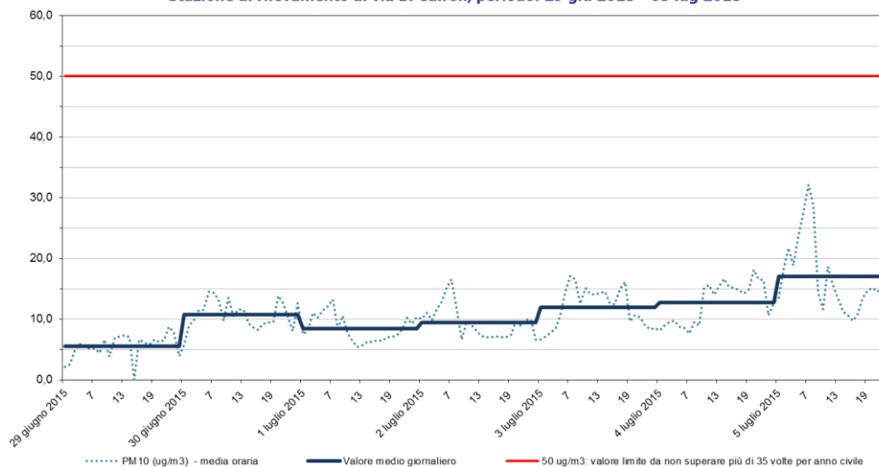
PM10 Stazione di rilevamento di via B. Cairoli, periodo: 29 giu 2015 - 05 lug 2015
