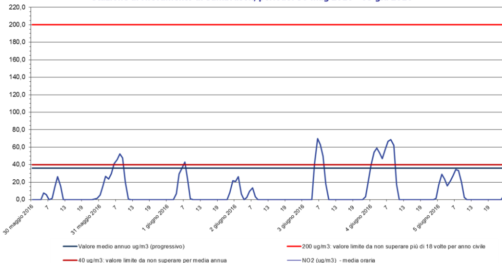
Biossido di azoto - NO 2 Stazione di rilevamento di Sambruson, periodo: 30 mag 2016 - 05 giu 2016
