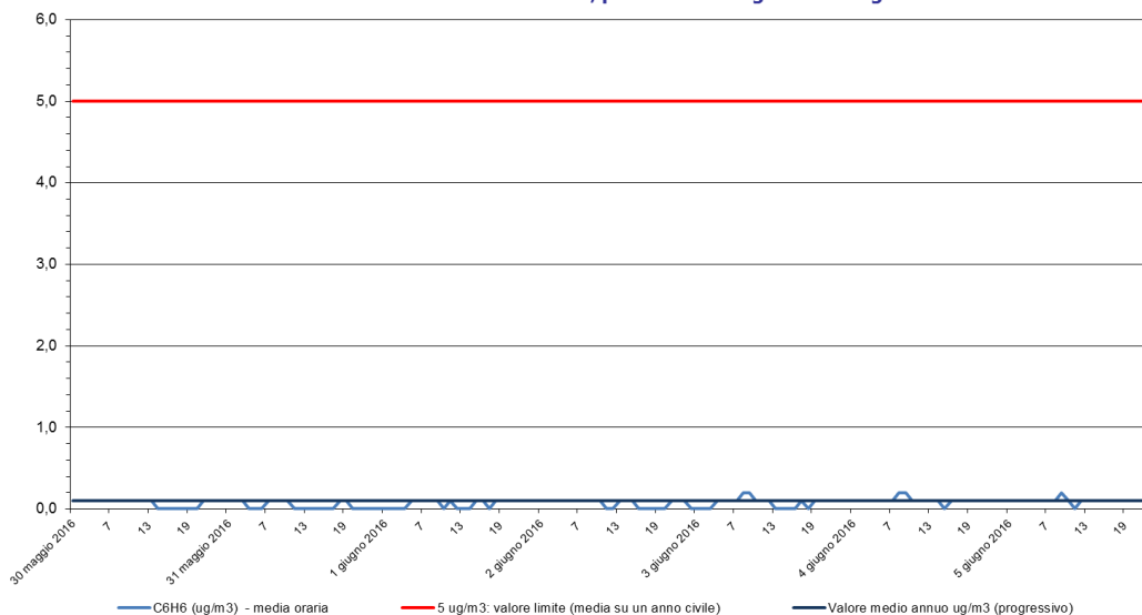
Benzene - C 6 H 6 Stazione di rilevamento di Sambruson, periodo: 30 mag 2016 - 05 giu 2016
