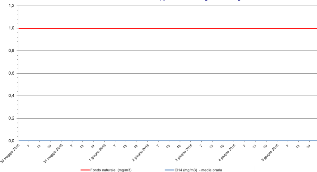
Metano - CH 4 Stazione di rilevamento di Sambruson, periodo: 30 mag 2016 - 05 giu 2016
