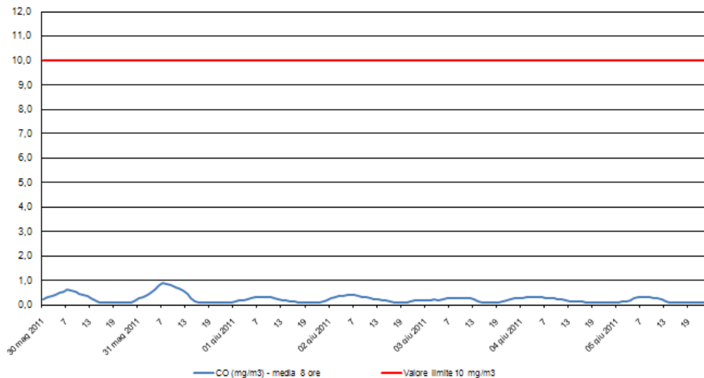
Monossido di Carbonio - CO Stazione di rilevamento di via B. Cairoli, periodo: 30 mag 2011 - 05 giu 2011
