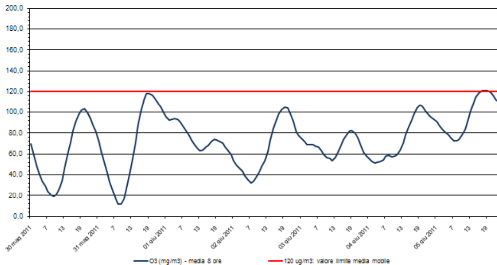
Ozono - O3 Stazione di rilevamento di via B. Cairoli, periodo: 30 mag 2011 - 05 giu 2011
