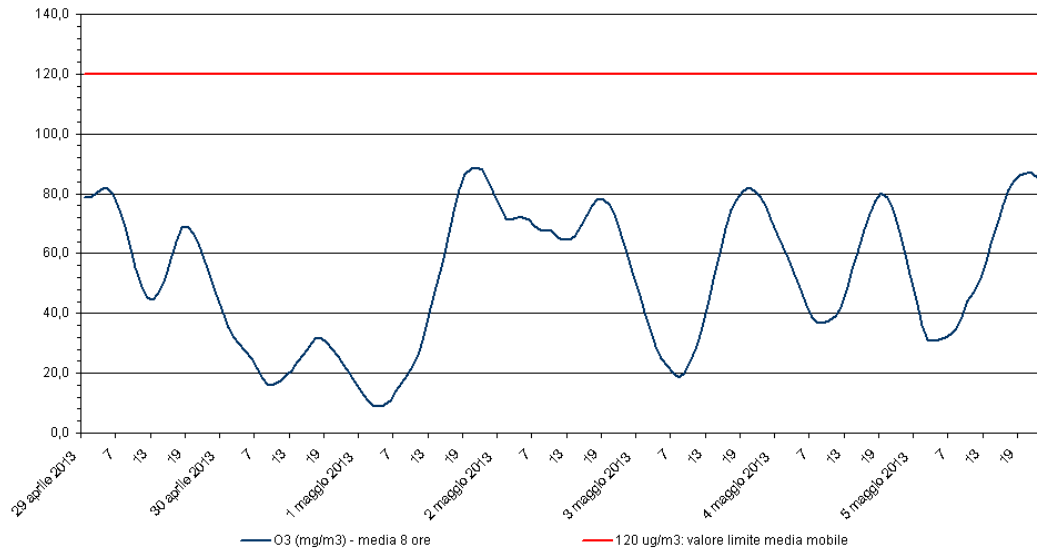
Ozono - O3 Stazione di rilevamento di Sambruson, periodo: 29 apr 2013 - 05 mag 2013
