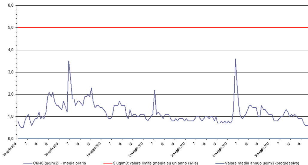
Benzene - C 6 H 6 Stazione di rilevamento di Sambruson, periodo: 29 apr 2013 - 05 mag 2013
