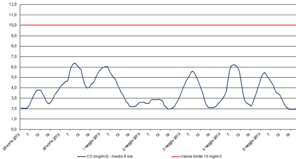
Monossido di Carbonio - CO Stazione di rilevamento di Sambruson, periodo: 29 apr 2013 - 05 mag 2013
