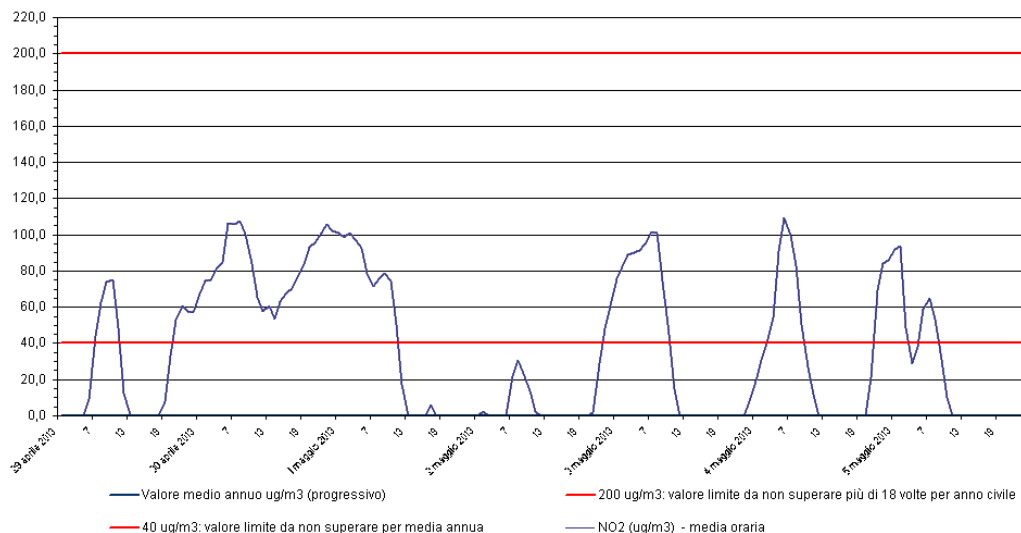
Biossido di azoto - NO 2 Stazione di rilevamento di Sambruson, periodo: 29 apr 2013 - 05 mag 2013
