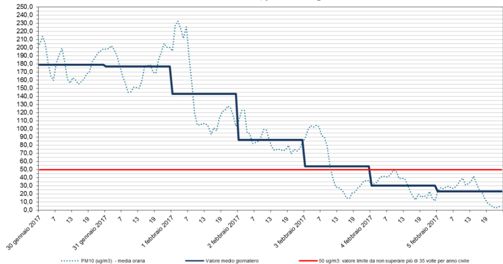
PM10 Stazione di rilevamento di via B. Cairoli, periodo: 30 gen 2017 - 05 feb 2017
