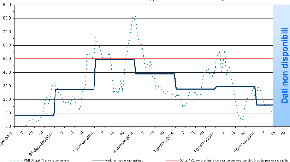
PM10 Stazione di rilevamento di via B. Cairoli, periodo: 30 dic 2013 - 05 gen 2014
