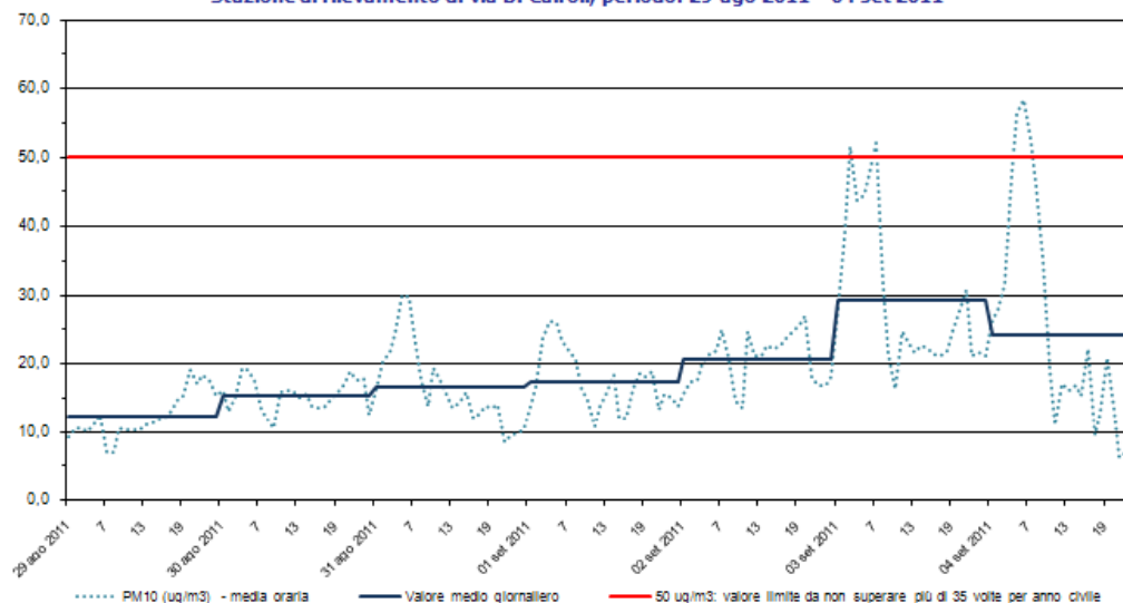
PM10 Stazione di rilevamento di via B. Cairoli, periodo: 29 ago 2011 - 04 set 2011
