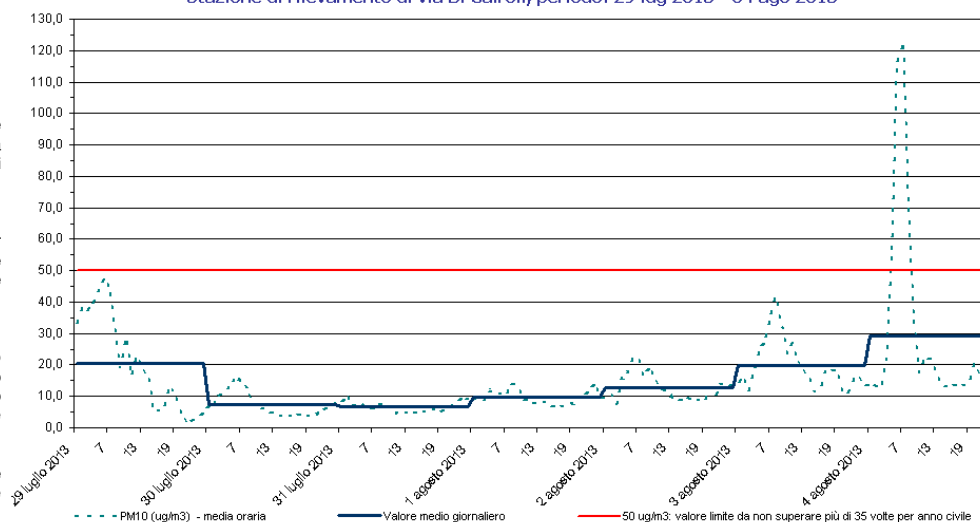
PM10 Stazione di rilevamento di via B. Cairoli, periodo: 29 lug 2013 - 04 ago 2013
