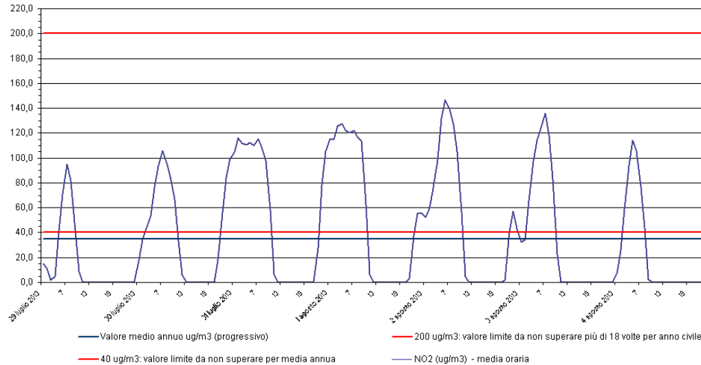
Biossido di azoto - NO 2 Stazione di rilevamento di Sambruson, periodo: 29 lug 2013 - 04 ago 2013
