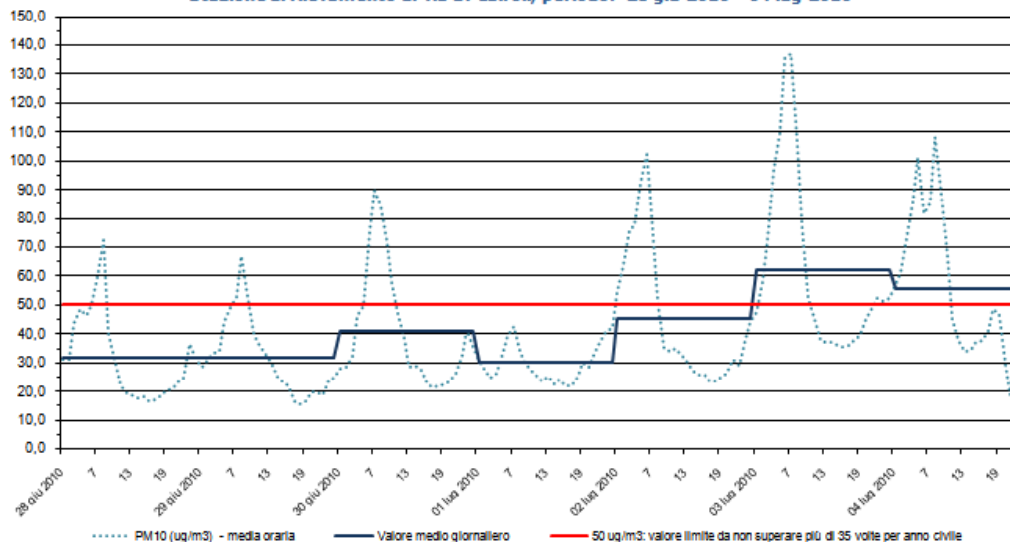
PM 10 Stazione di rilevamento di via B. Cairoli, periodo: 28 giu 2010 - 04 lug 2010
