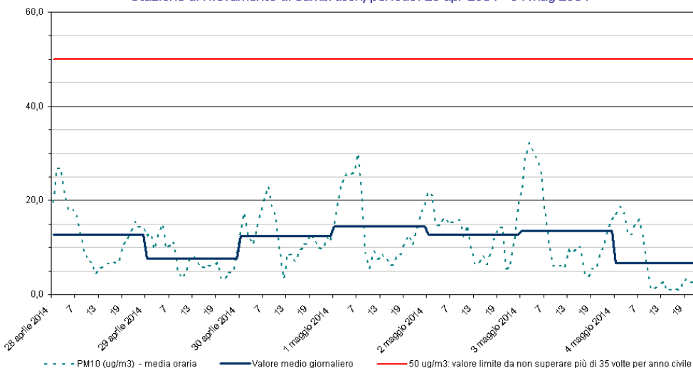
PM 10 Stazione di rilevamento di Sambruson, periodo: 28 apr 2014 - 04 mag 2014
