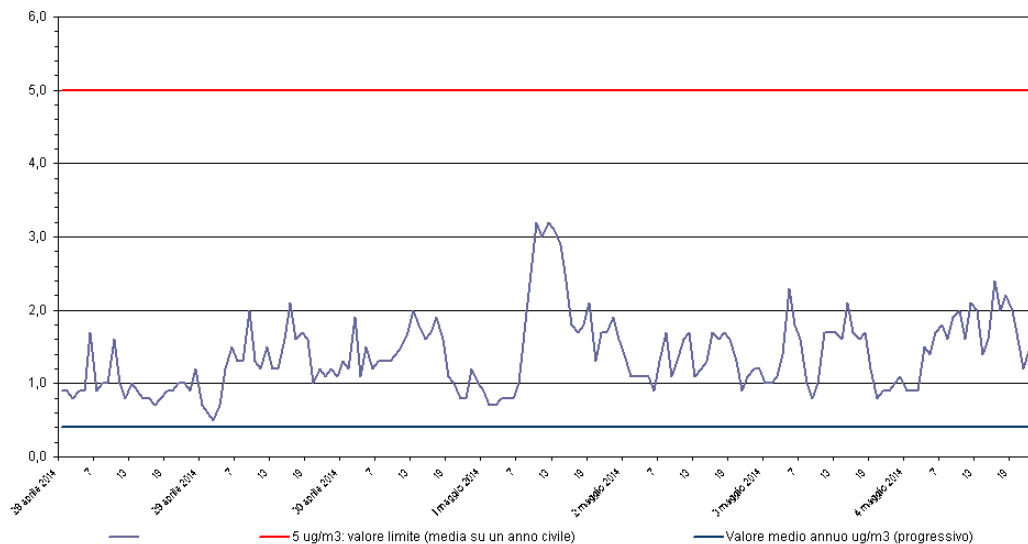
Benzene - C 6 H 6 Stazione di rilevamento di Sambruson, periodo: 28 apr 2014 - 04 mag 2014
