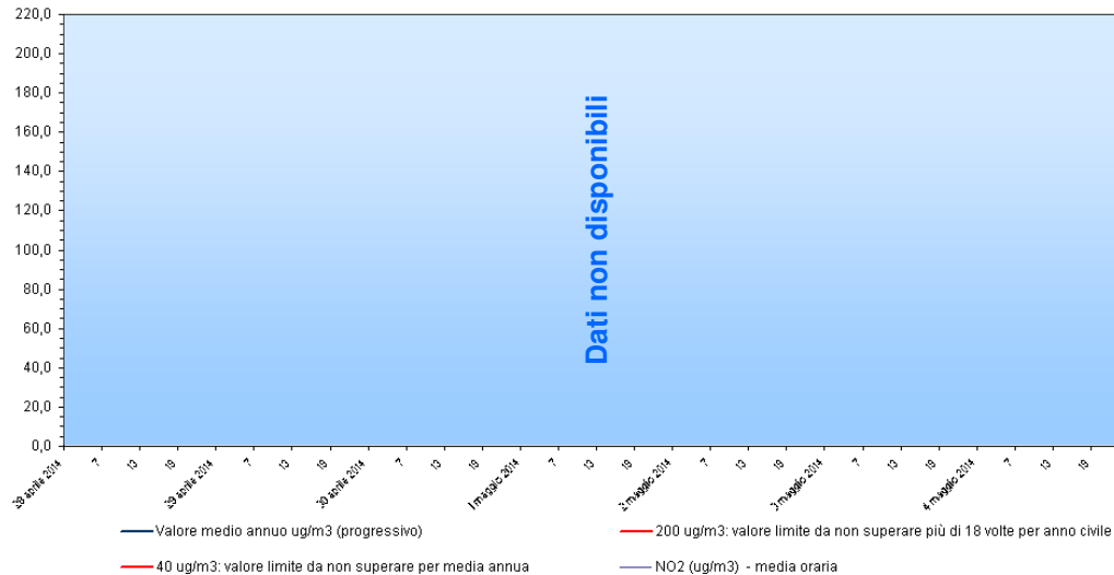
Biossido di azoto - NO 2 Stazione di rilevamento di Sambruson, periodo: 28 apr 2014 - 04 mag 2014
