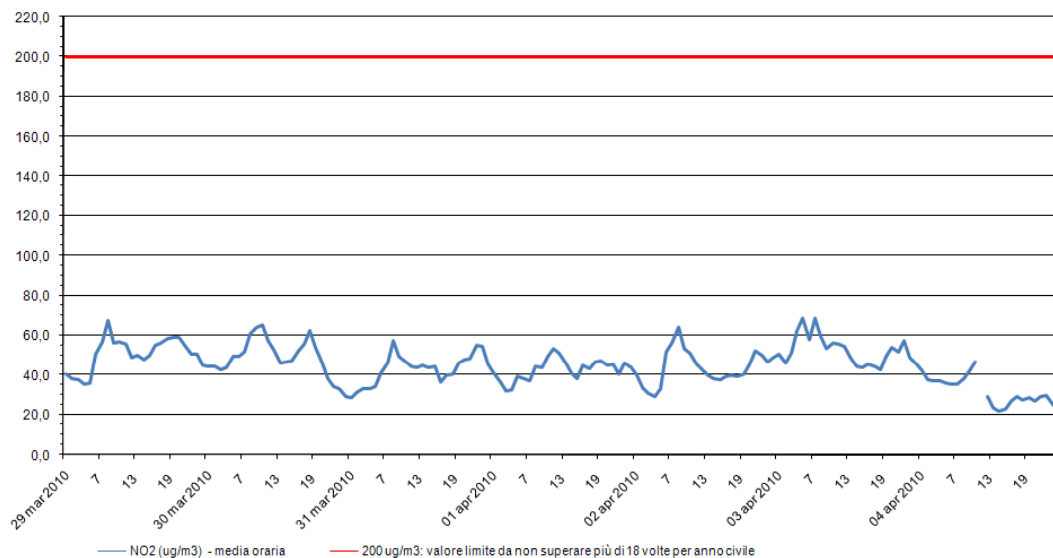
Biossido di azoto - NO 2 Stazione di rilevamento di via B. Cairoli, periodo: 29 mar 2010 - 04 apr 2010
