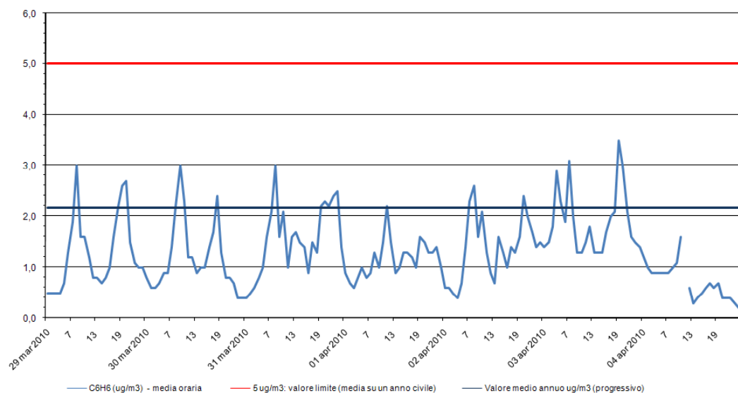
Benzene - C 6 H 6 Stazione di rilevamento di via B. Cairoli, periodo: 29 mar 2010 - 04 apr 2010
