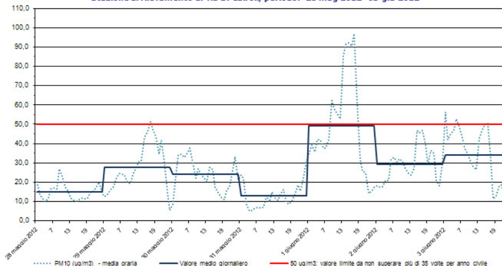
PM10 Stazione di rilevamento di via B. Cairoli, periodo: 28 mag 2012- 03 giu 2012
