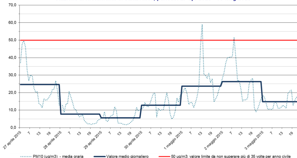
PM10 Stazione di rilevamento di Sambruson, periodo: 27 apr 2015 - 03 mag 2015
