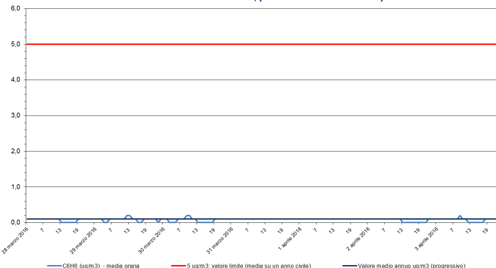
Benzene - C 6 H 6 Stazione di rilevamento di Sambruson, periodo: 28 mar 2016 - 03 apr 2016
