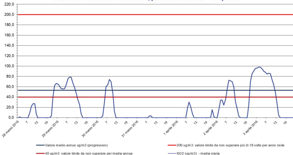
Biossido di azoto - NO 2 Stazione di rilevamento di Sambruson, periodo: 28 mar 2016 - 03 apr 2016
