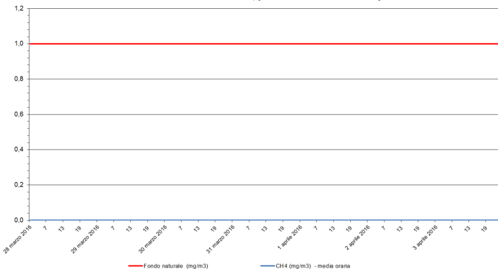
Metano - CH 4 Stazione di rilevamento di Sambruson, periodo: 28 mar 2016 - 03 apr 2016
