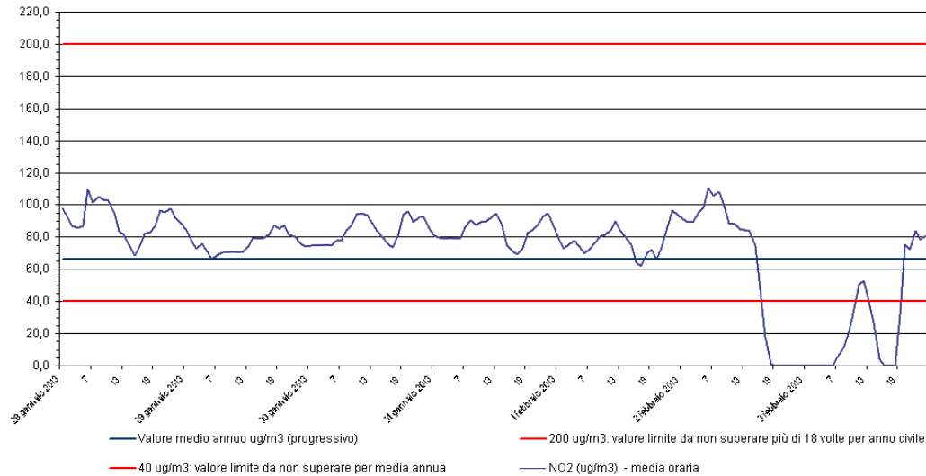
Biossido di azoto - NO 2 Stazione di rilevamento di Sambruson, periodo: 28 gen 2013 - 03 feb 2013
