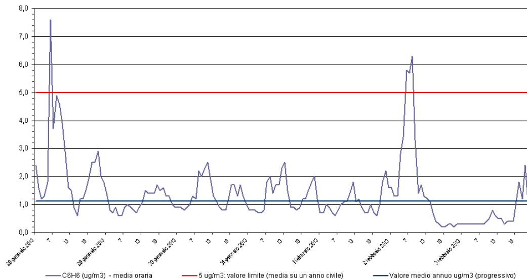
Benzene - C 6 H 6 Stazione di rilevamento di Sambruson, periodo: 28 gen 2013 - 03 feb 2013
