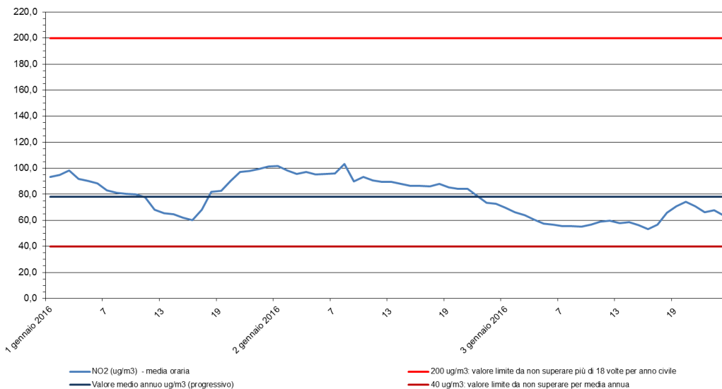
Biossido di azoto - NO 2 Stazione di rilevamento di via B. Cairoli, periodo: 01 gen 2016 - 03 gen 2016
