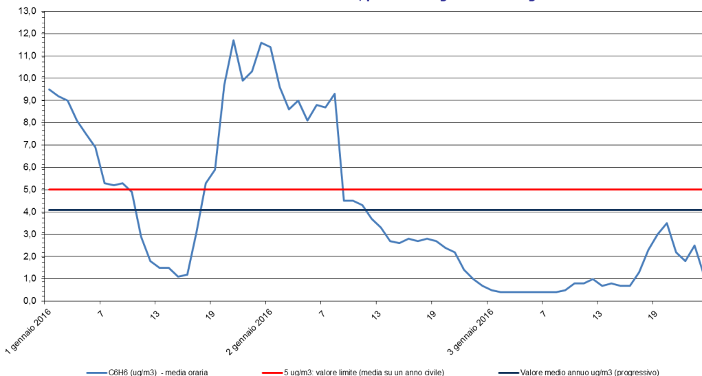
Benzene - C 6 H 6 Stazione di rilevamento di via B. Cairoli, periodo: 01 gen 2016 - 03 gen 2016
