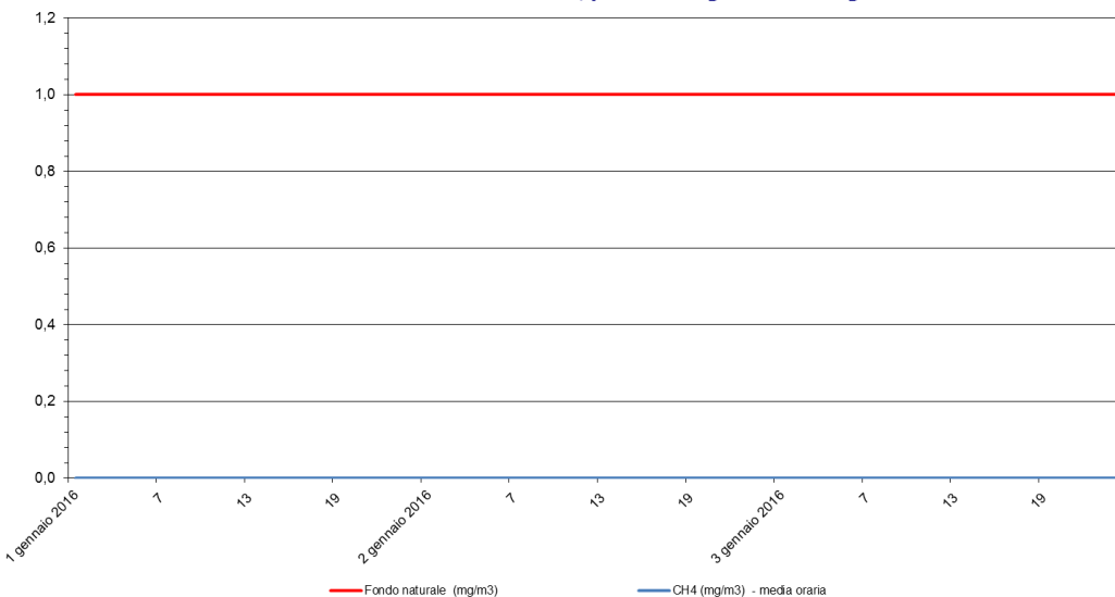
Metano - CH 4 Stazione di rilevamento di via B. Cairoli, periodo: 01 gen 2016 - 03 gen 2016
