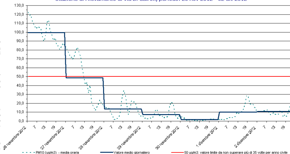
PM 10 Stazione di rilevamento di via B. Cairoli, periodo: 26 nov 2012 - 02 dic 2012
