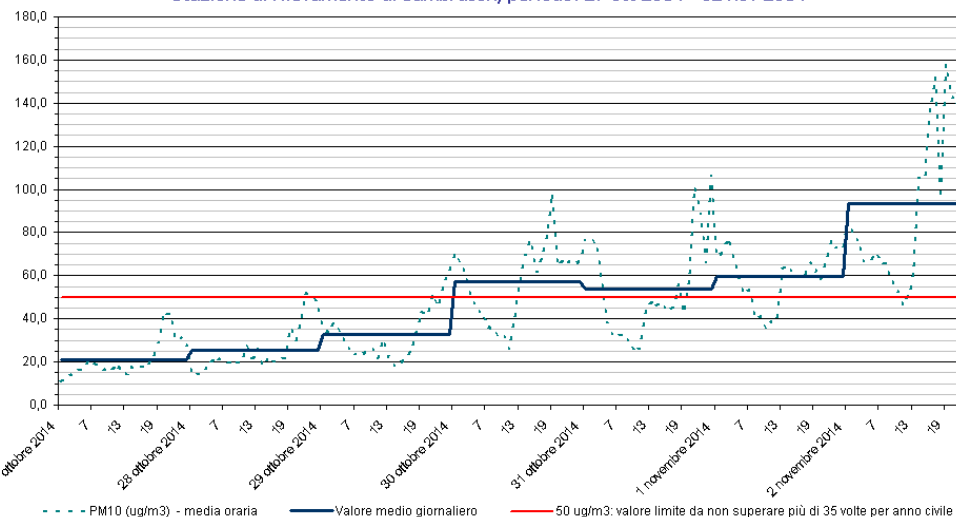
PM10 Stazione di rilevamento di Sambruson, periodo: 27 ott 2014 - 02 nov 2014
