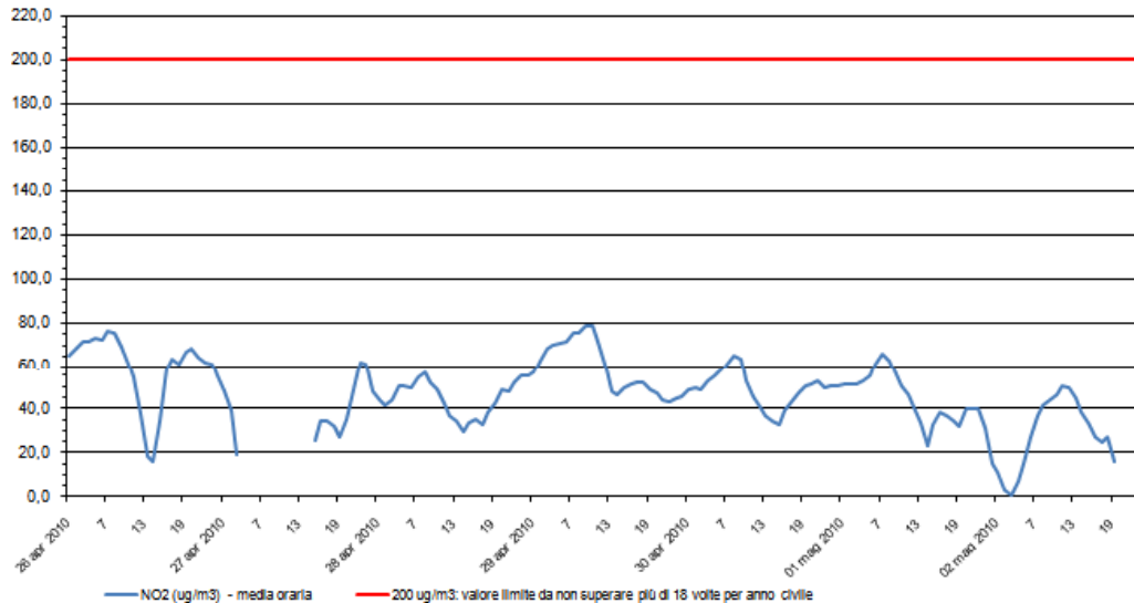
Biossido di azoto - NO 2 Stazione di rilevamento di via F.lli Bandiera, periodo: 26 apr 2010 - 02 mag 2010
