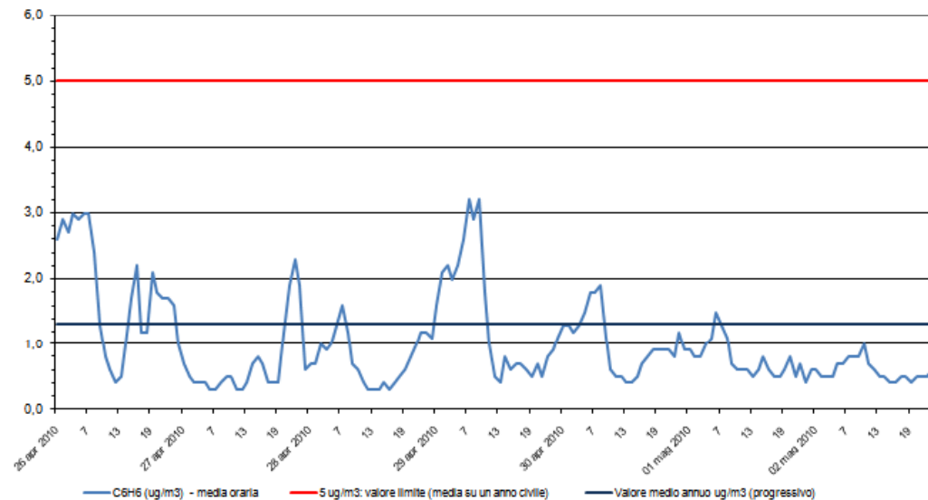
Benzene - C 6 H 6 Stazione di rilevamento di via F.lli Bandiera, periodo: 26 apr 2010 - 02 mag 2010
