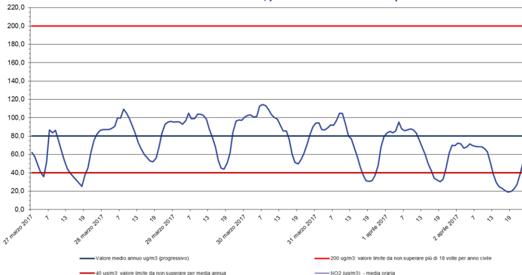
Biossido di azoto - NO 2 Stazione di rilevamento di Sambruson, periodo: 27 mar 2017 - 02 apr 2017
