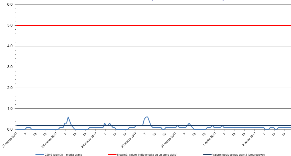
Benzene - C 6 H 6 Stazione di rilevamento di Sambruson, periodo: 27 mar 2017 - 02 apr 2017
