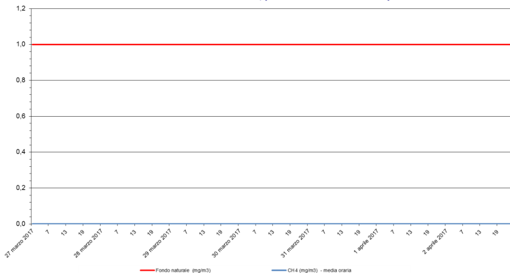
Metano - CH 4 Stazione di rilevamento di Sambruson, periodo: 27 mar 2017 - 02 apr 2017
